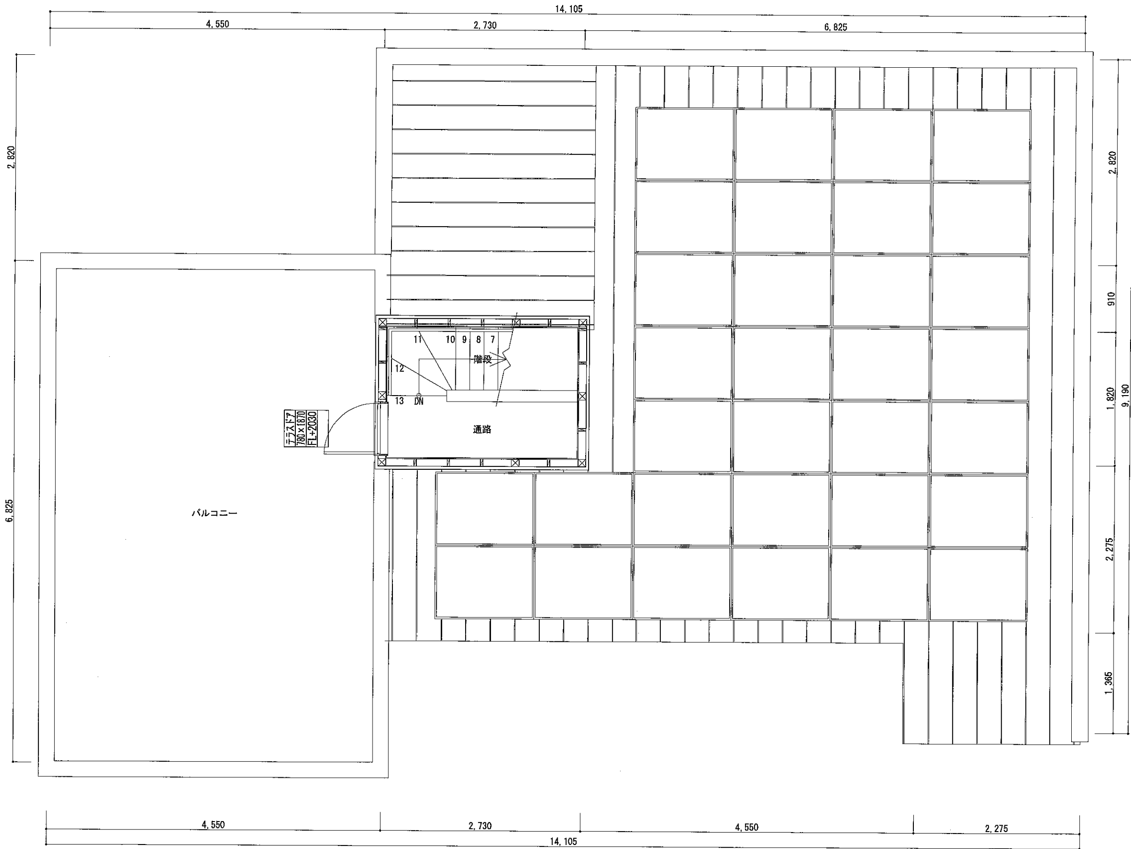
PH階 平面詳細図 S:1/50
